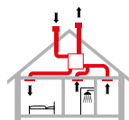
Ventilation contrôlée de l'habitation (VMC)
